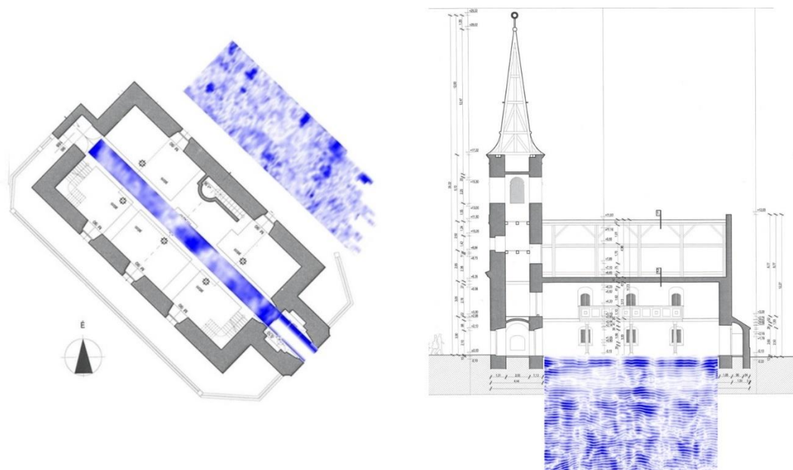
13. ábra A mihályházi református templom alaprajzára és metszetére vetített mérés képei. A felmérést végezte Györffy-Villám Zsombor - Pátkai Ádám Sándor, az építészeti felmérést Mezei László végezte.
