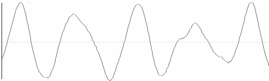
Abb. 8 Komplexe Schallwelle - die Schwingungsperiode eines Gitarrenklangs
